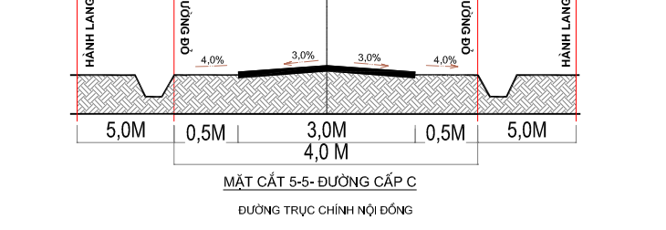
MẶT CẮT 5-5: ĐƯỜNG CẤP C
