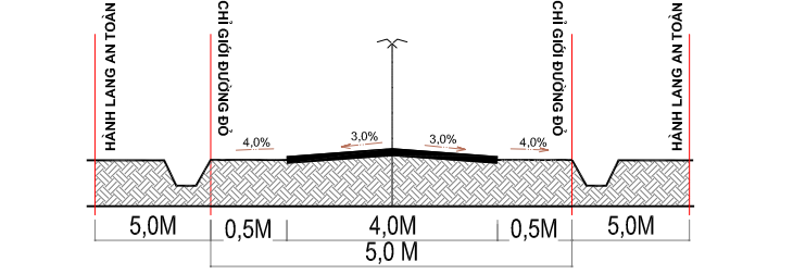
MẶT CẮT 4-4: ĐƯỜNG CẤP B
