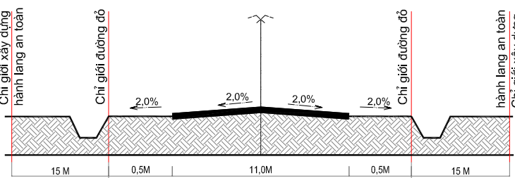
MẶT CẮT 1:1: QUỐC LỘ 3
