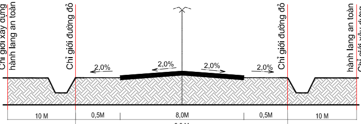
MẶT CẮT 1B-1B: QUỐC LỘ 3C
