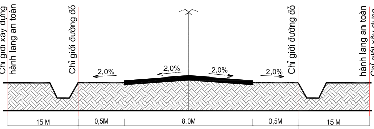
MẶT CẮT 1C-1C: ĐƯỜNG VÀNH ĐAI 2
