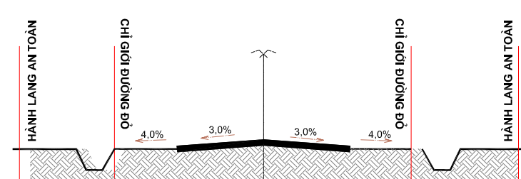
MẶT CẮT 2-2: ĐƯỜNG CẤP BÙ MỀM NHỎ
